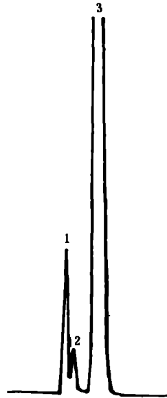
图 2 溴甲烷原药气相色谱图(面积归一法) 1—甲醚;2—氯甲烷;3—溴甲烷
